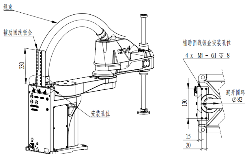
图 5-5 线缆走线示意图
