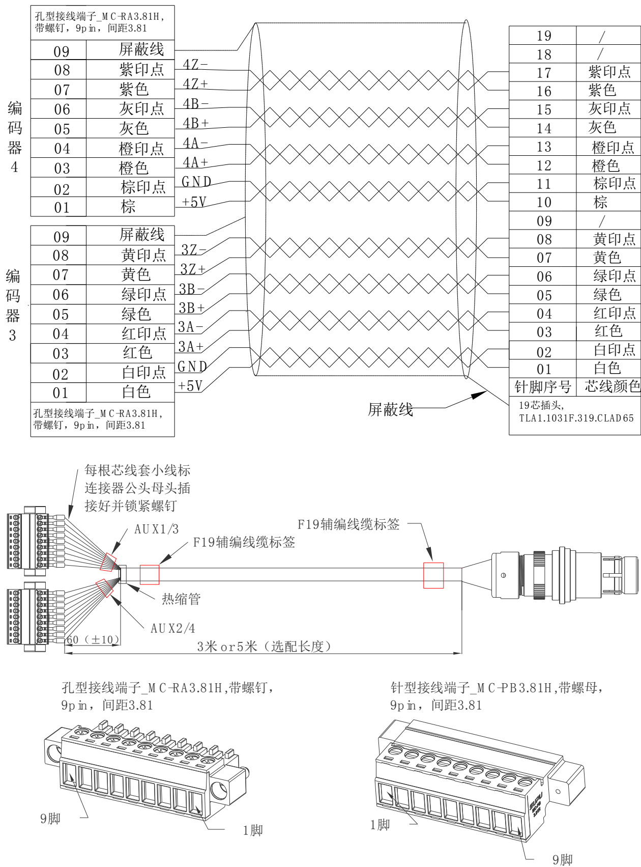
图 4-5 辅助编码器选配线
