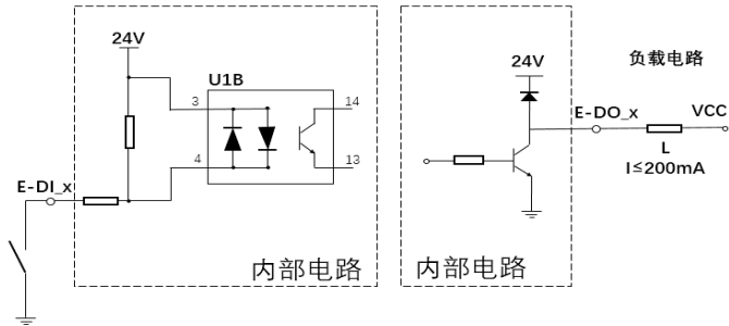
图 4-7 输入电路图（左）和输出电路图（右）
