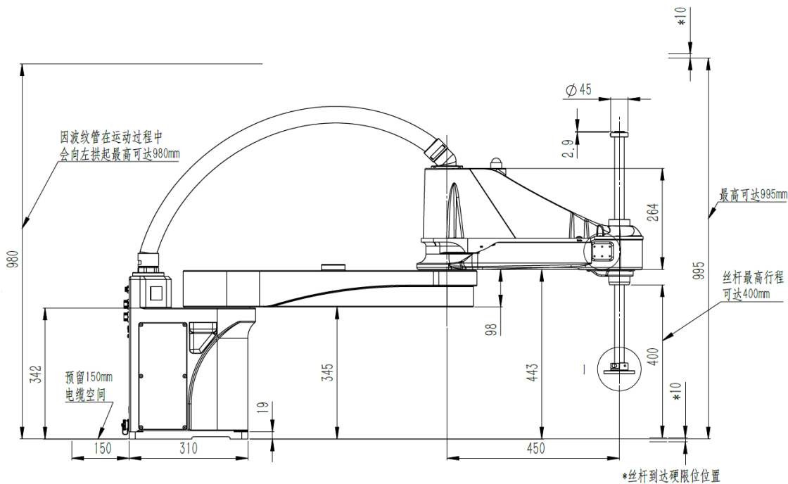
图 3-13 AH20-1050-0204-4000 的产品尺寸图（单位：mm）
