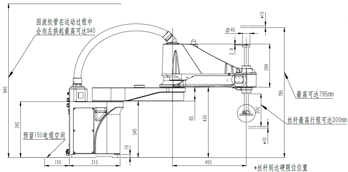
图 3-7 AH20-0850-0204-2000 的产品尺寸图 (单位: mm)
