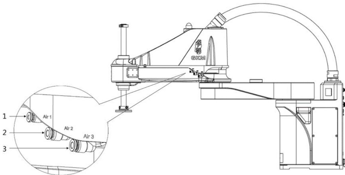
图 4-2 接气孔示意图
