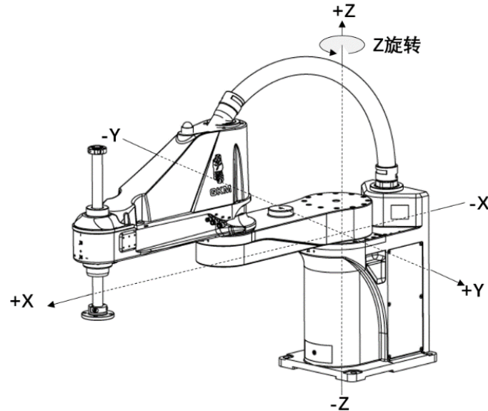
图 3-6 世界坐标系
