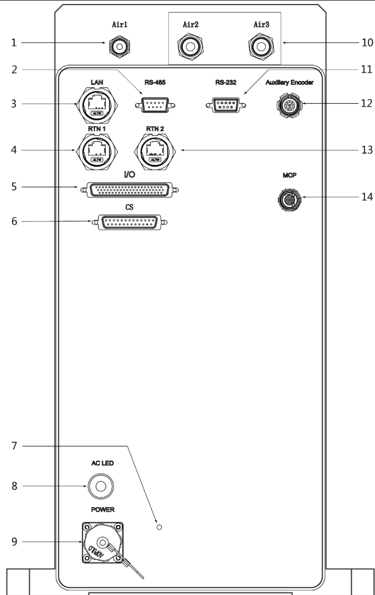
图 4-4 接口面板示意图
