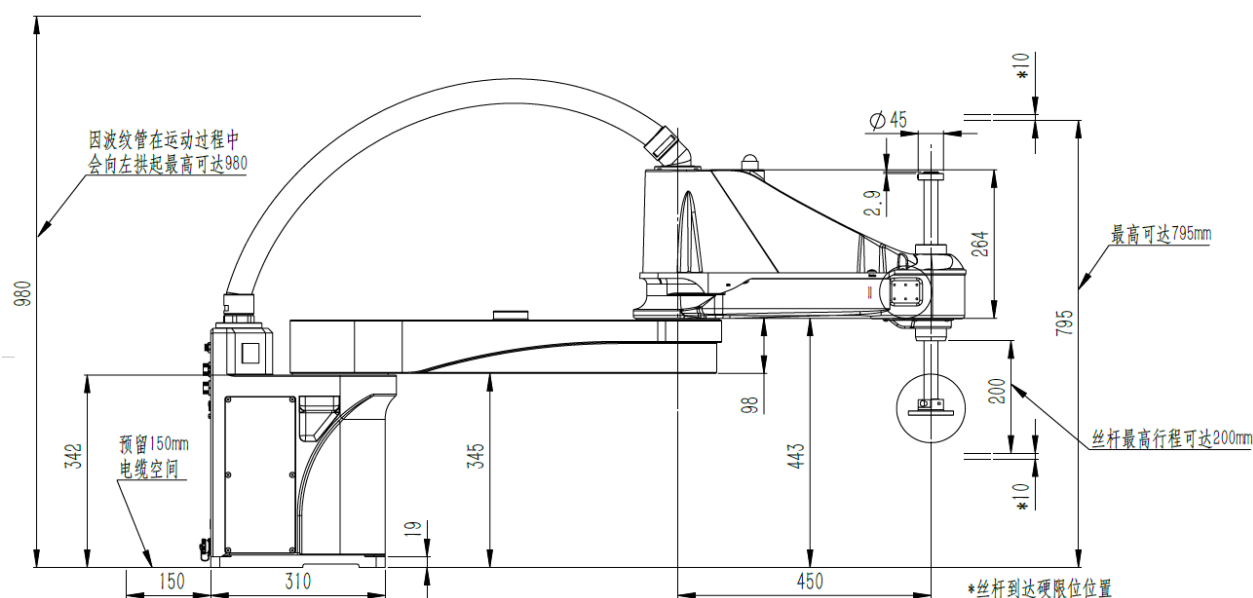
图 3-11 AH20-1050-0204-2000 的产品尺寸图 (单位: mm)
