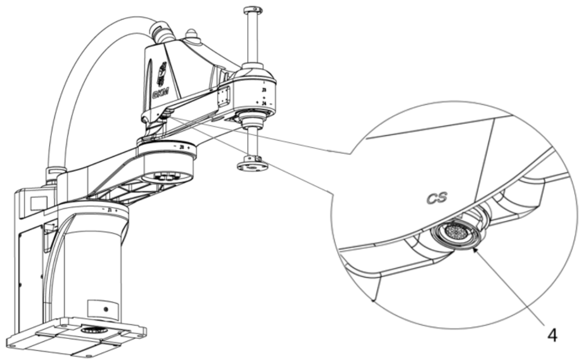
图 4-3 CS 接口示意图
