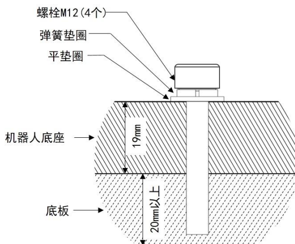
图 5-2 安装示例图
