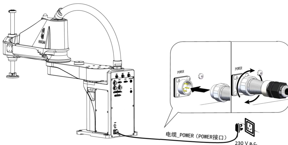
图 5-12 连接电源
