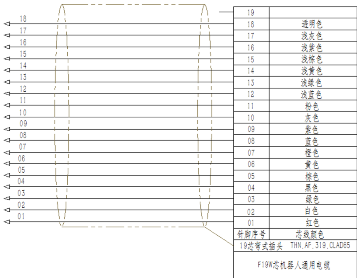
图 4-8 F19W 芯机器人通用电缆连接图
