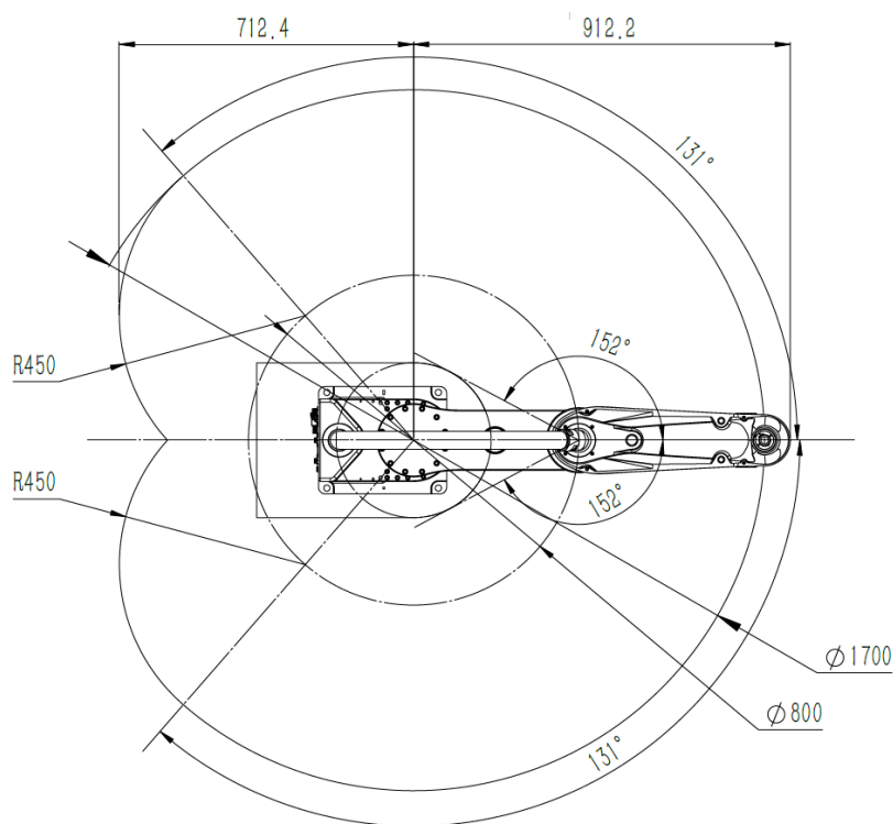
图 3-4 AH20-0850-0204-2000 / AH20-0850-0204-4000
