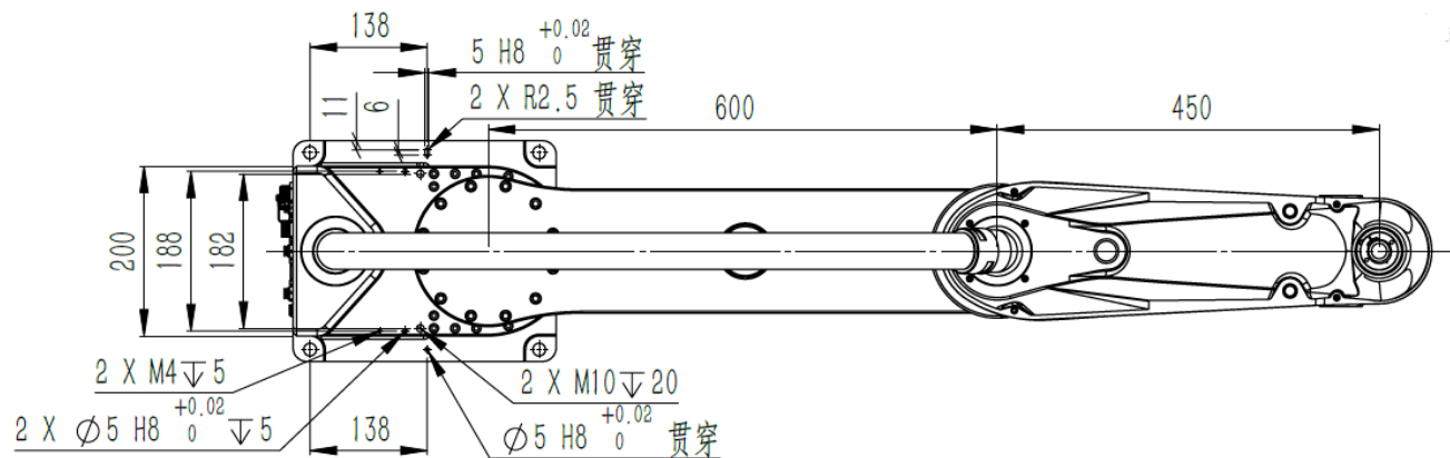
图 3-14 AH20-1050-0204-4000 的产品尺寸图（单位：mm）
