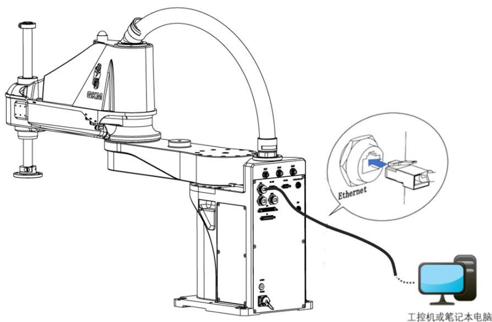
图 5-10 通讯连接示意图
