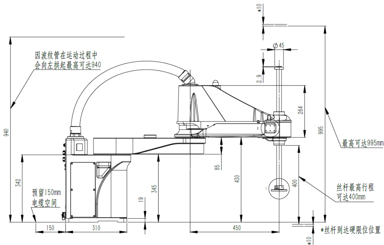
图 3-9 AH20-0850-0204-4000 的产品尺寸图（单位：mm）
