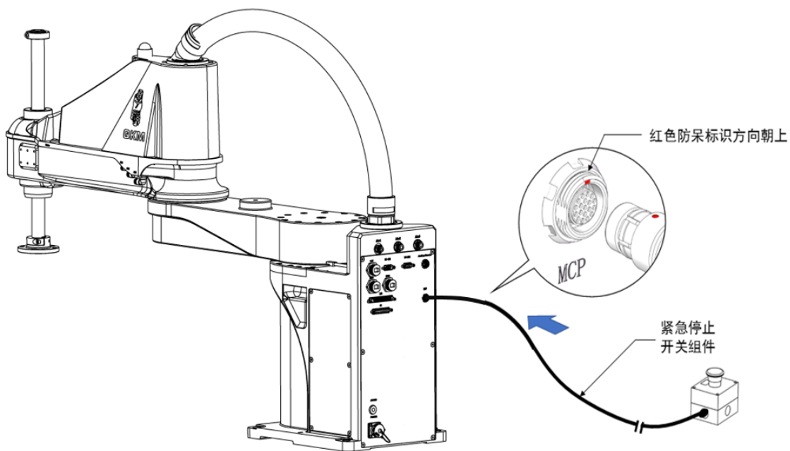
图 5-11 急停装置连接示意图
