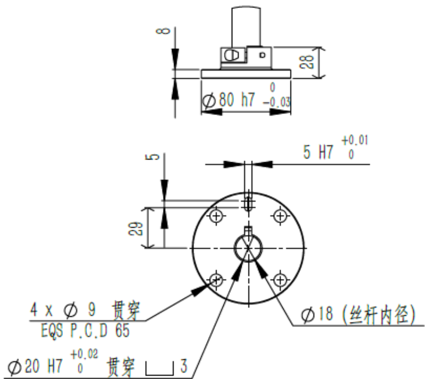
图 3-16 末端法兰安装尺寸图（单位：mm）
