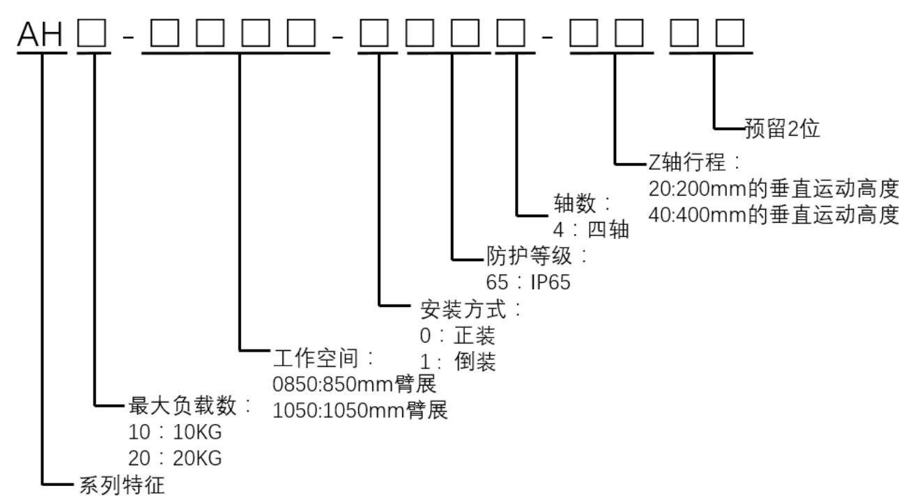
图 2-2 型号说明
