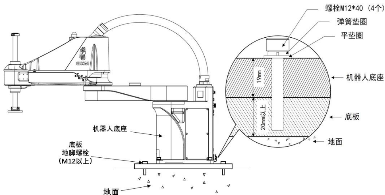
图 5-7 安装基座螺栓
