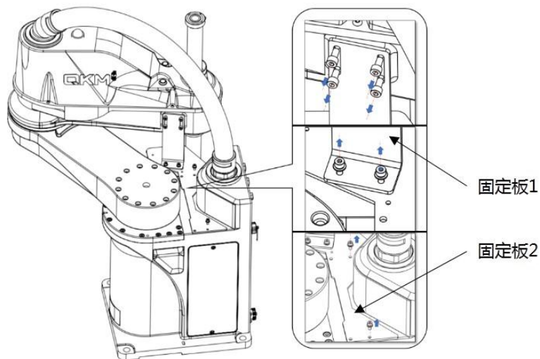
图 5-8 拆除固定板示意图
