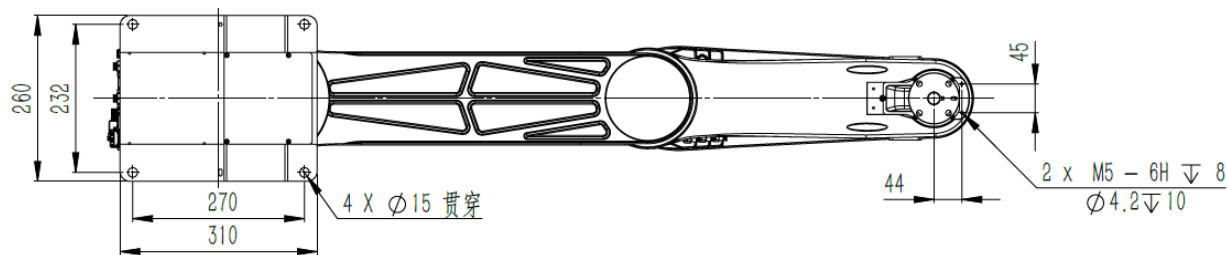
图 3-15 产品尺寸图（单位：mm）
