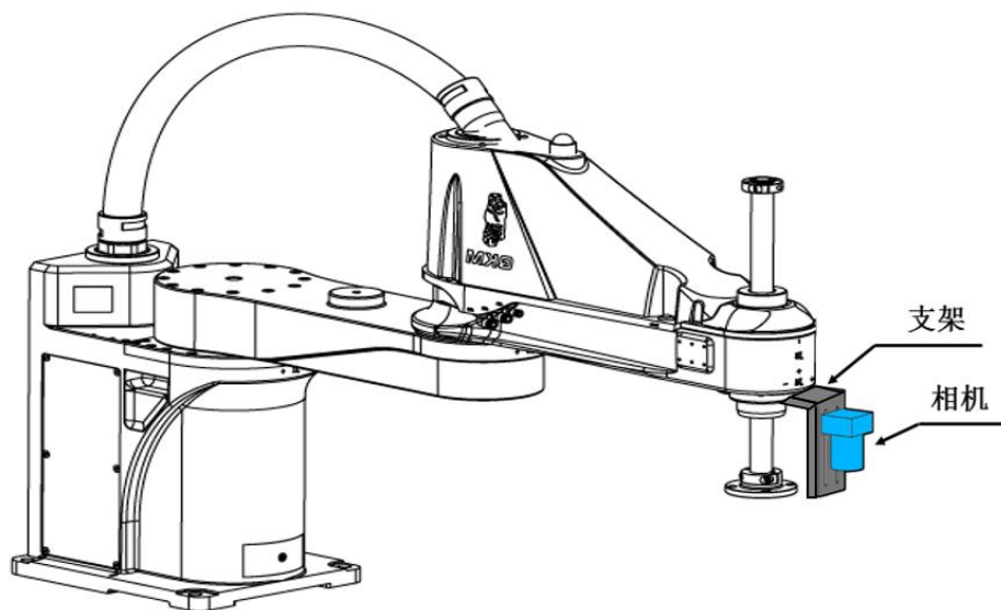
图 5-4 相机安装示意图
