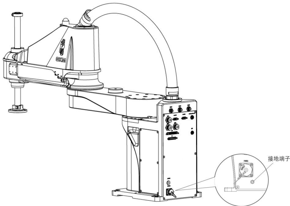
图 5-9 接地示意图
