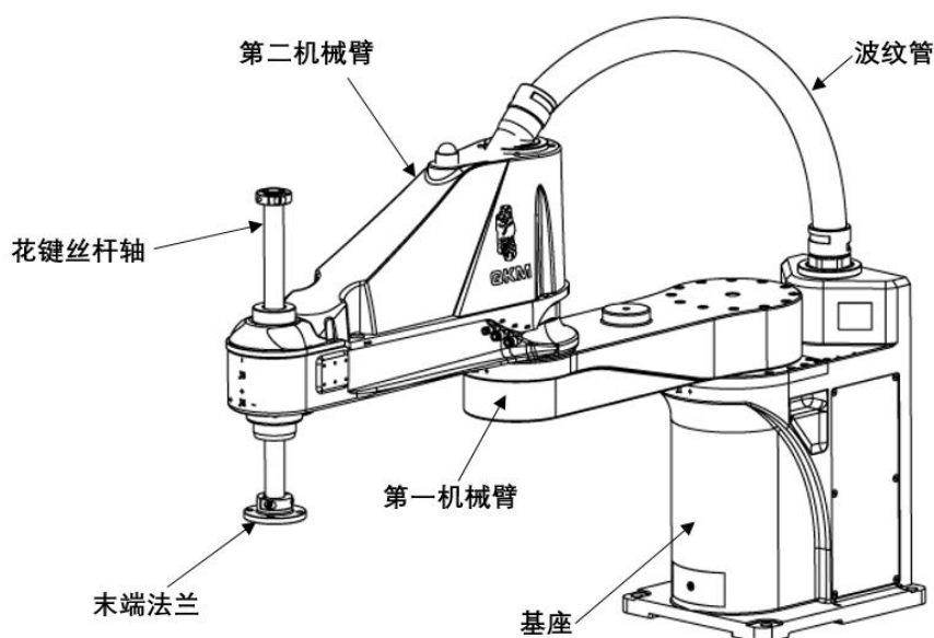
图 3-1 AH20 (AH20-0850-0204-2000) 机器人构成
