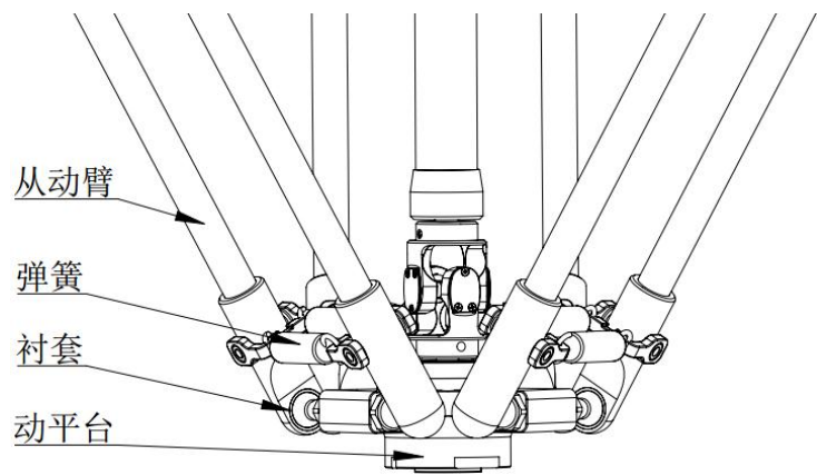
图 3-4 动平台与从动臂连接
