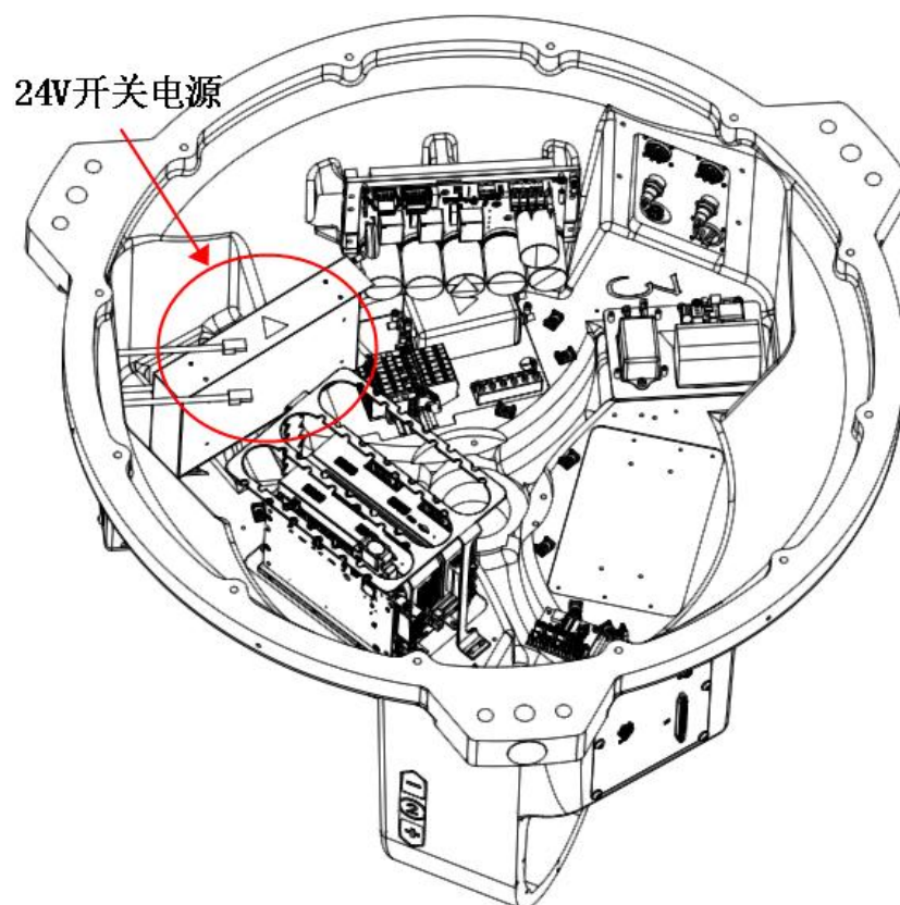
图 4-18 24V 开关电源位置示意图
