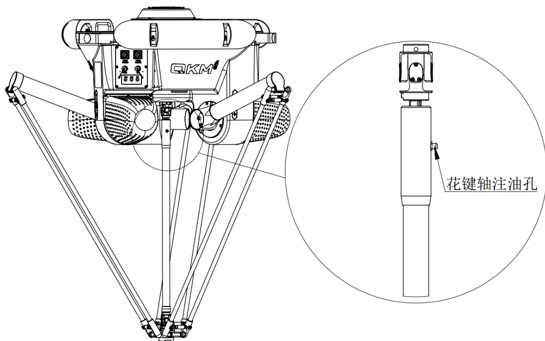
图 3-19 花键轴润滑
