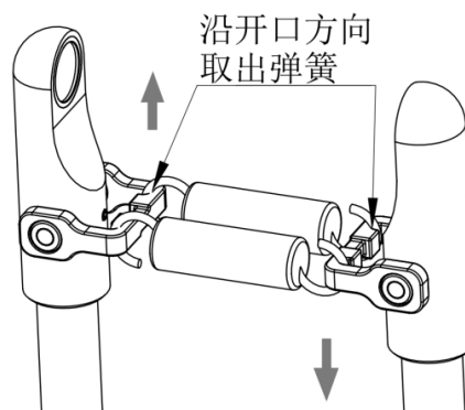
图 3-18 取出弹簧
