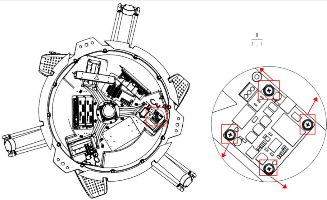
图 4-22 拆卸 UPS 电源 PCBA 固定螺钉
