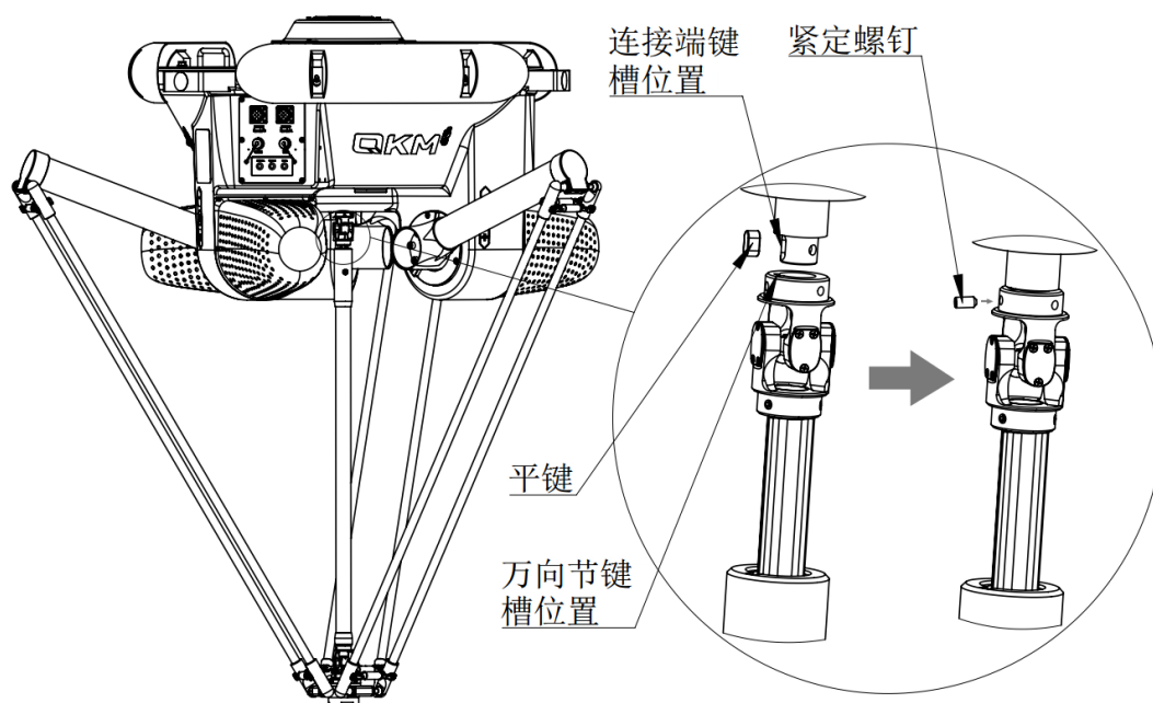
图 3-15 插入万向节
