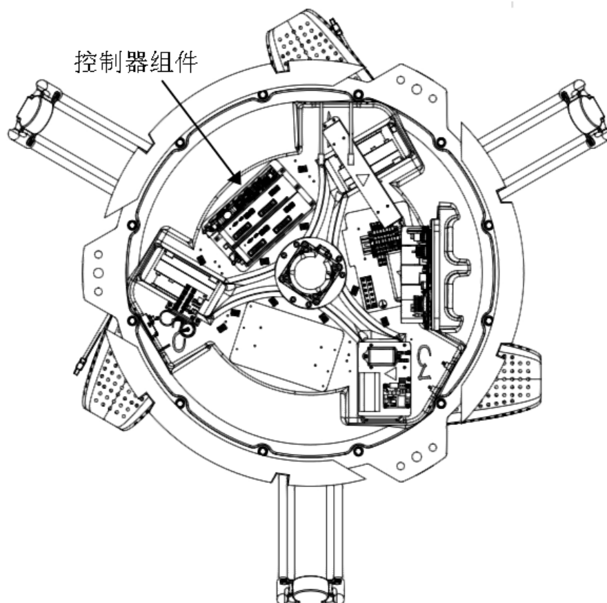
图 4-5 控制器示意图
