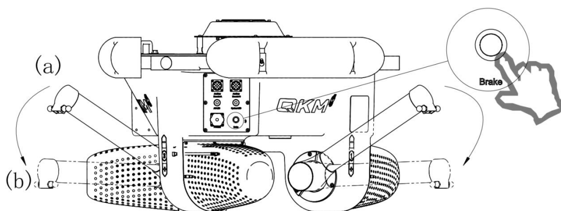
图 3-5 调整主动臂位置
