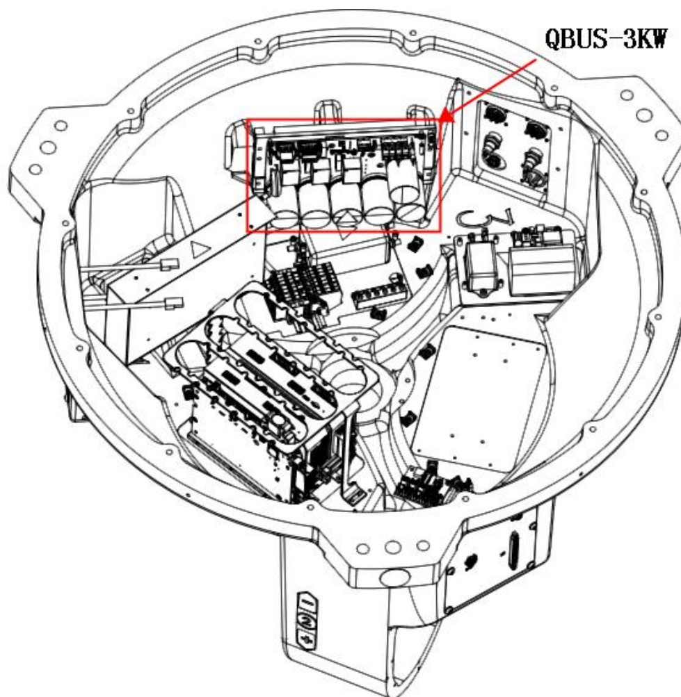
图 4-16 QBUS-3kW 位置示意图
