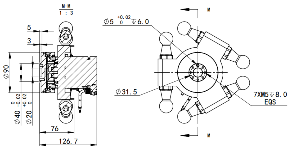
(b) 四轴动平台输出轴端法兰尺寸
