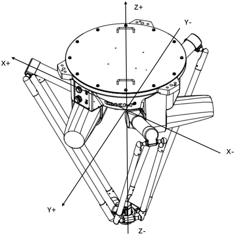
图 2-6 世界坐标系
