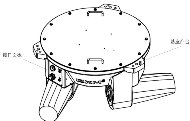
(a) 基座示意图
