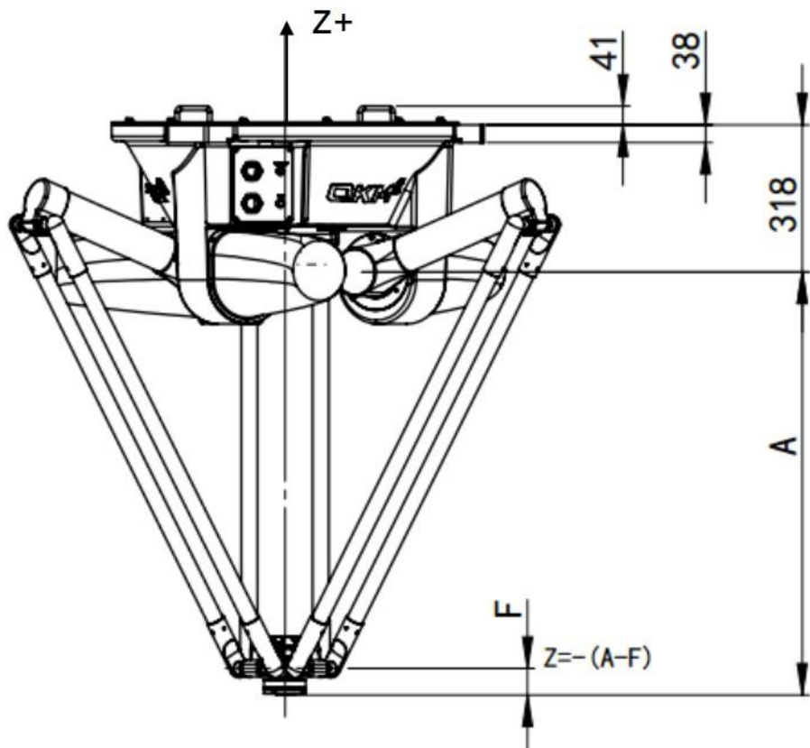
图 2-3 机器人整体尺寸
