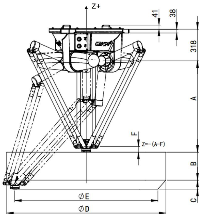
图 2-4 机器人工作空间主视图
