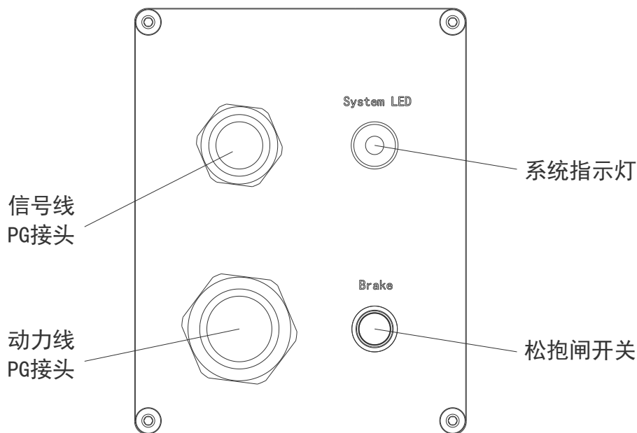
图 4-1 接口面板
