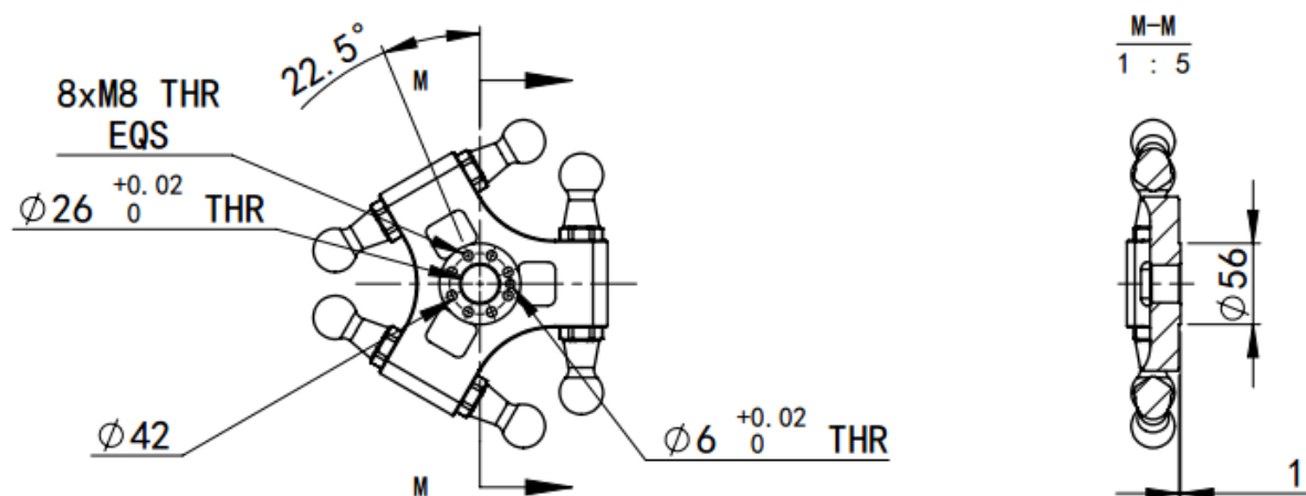
(a) 三轴动平台输出轴端法兰尺寸
