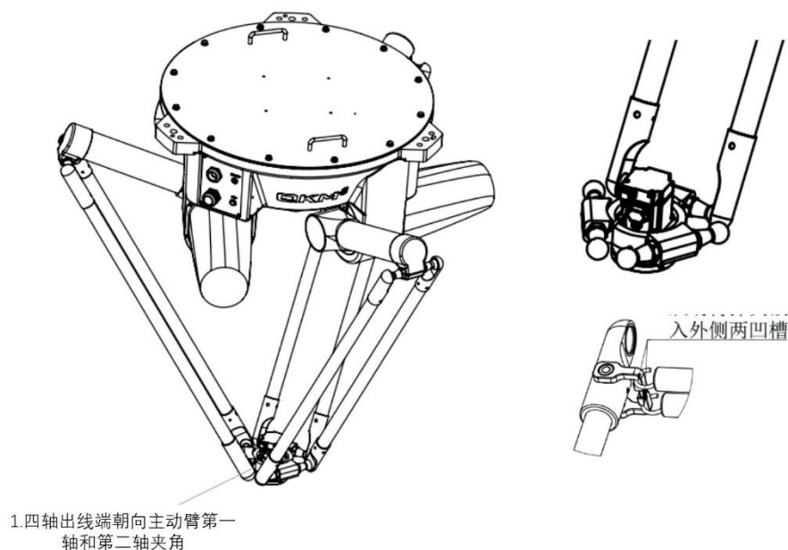
图 5-17 安装四轴机器人动平台旋转轴
