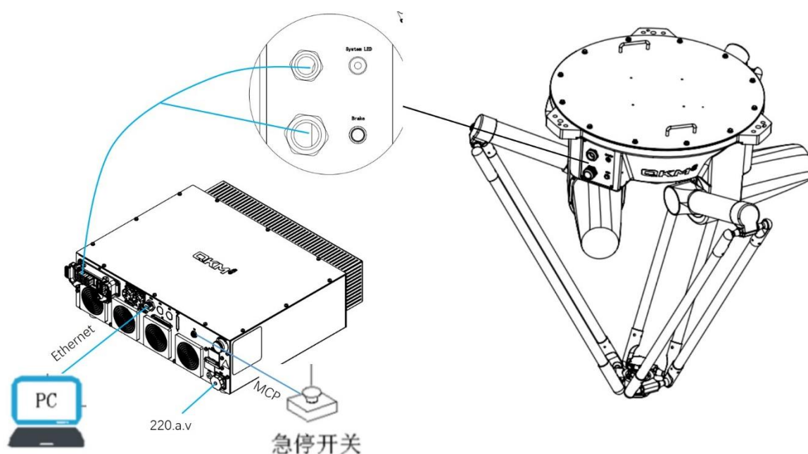
图 5-18 线缆安装示意图
