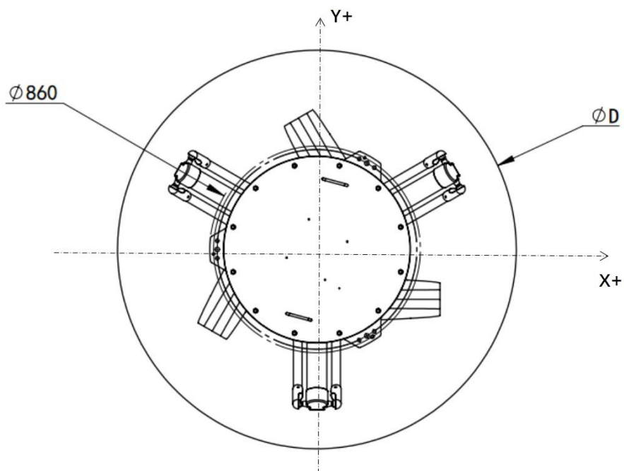
图 2-5 机器人工作空间俯视图
