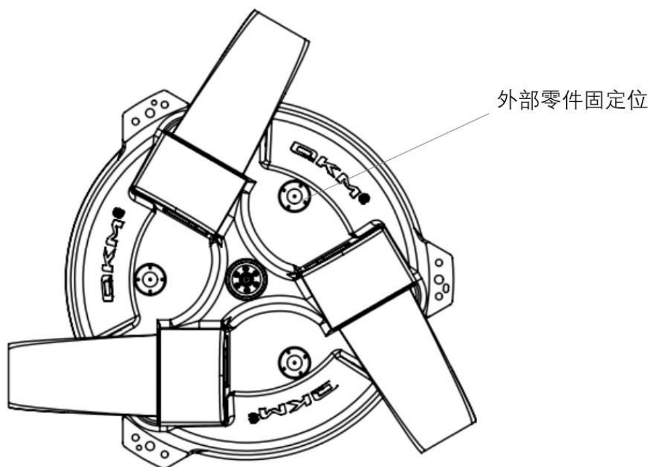
(a) 基座示意图
