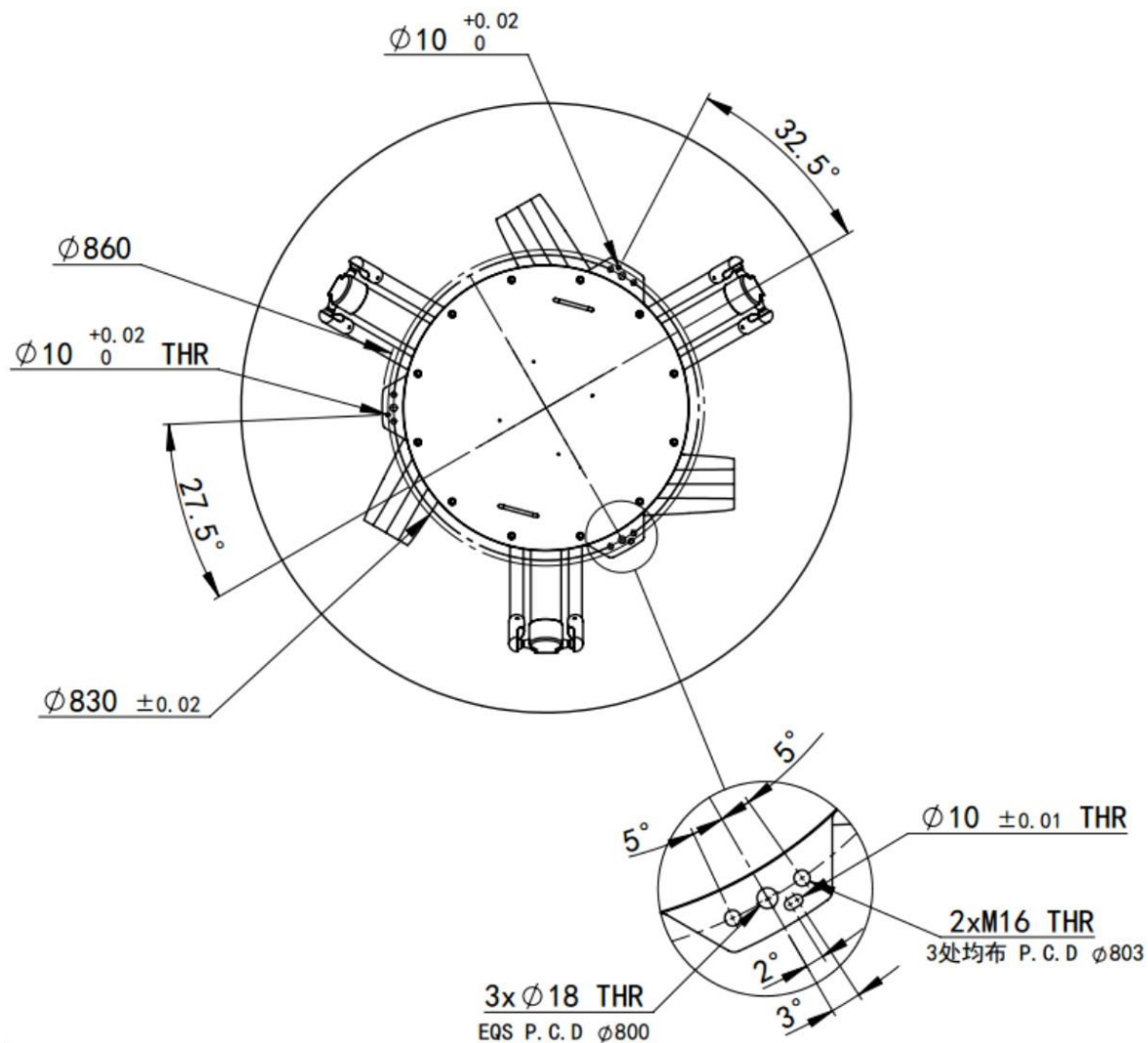
(c) 基座俯视图与局部视图尺寸
